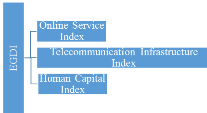
Рисунок 1 - Субіндекси EGDI.
